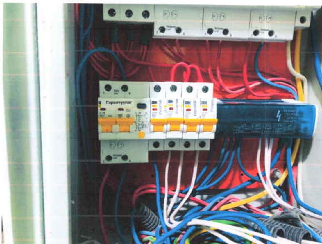
Барилгын дотор цахилгааны шийтэнд бирк хийж зааварчилгаа өгсөн
