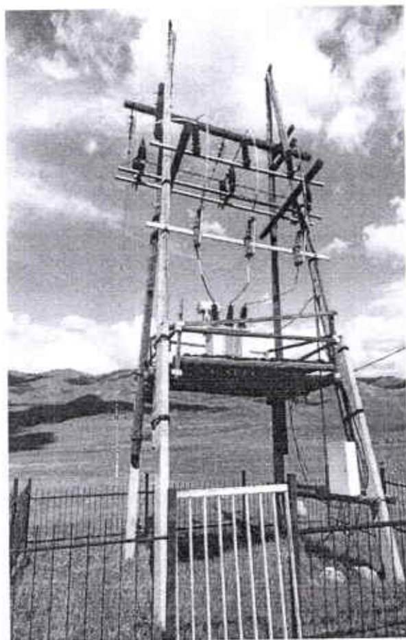
Иргэн О.Дашнямын 35/0,4кВ-н 250кВА чадал бүхий дэд өртөөнд өргөтгөл хийгдсэн нь:
