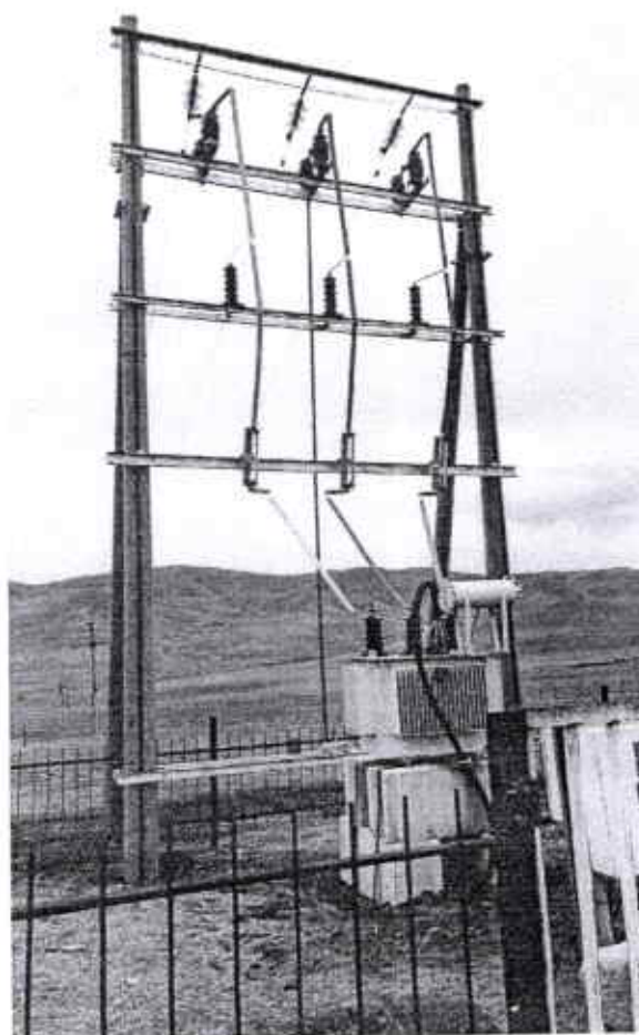
Иргэн О.Дашнямын 35/0,4кВ-н 250кВА чадал бүхий дэд өртөөнд өргөтгөл хийгдсэн нь:
