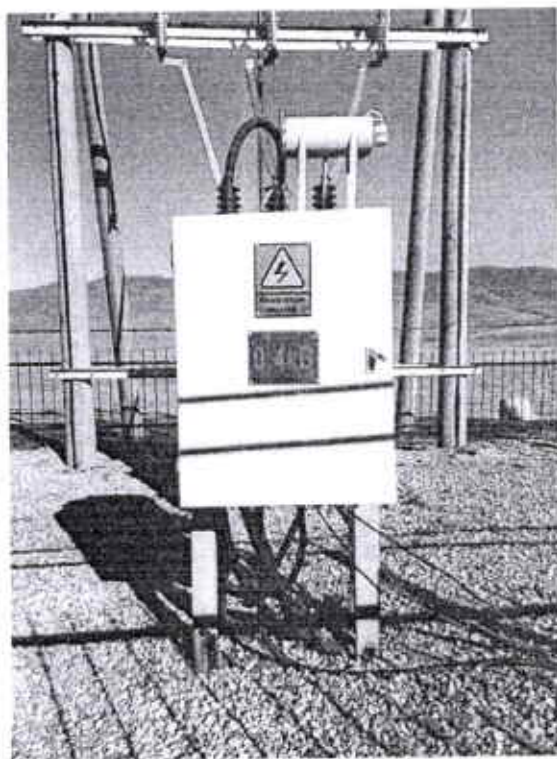
Дэд өртөөний хашаанд хайрга дэвссэн
